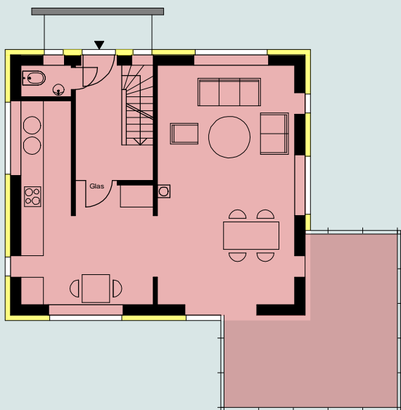
EG VARIANTE 2-Personenhaushalt
